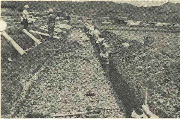
(写真) 若佐市街水道工事 中国附近本管工事
