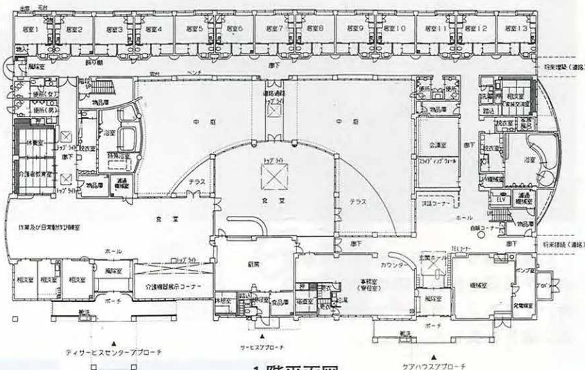
1階平面図
