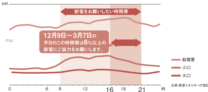
■冬の電気の使われ方（イメージ）
