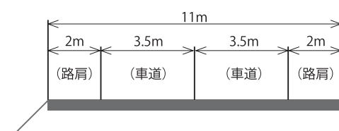
計画横断面
