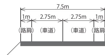
計画横断面
